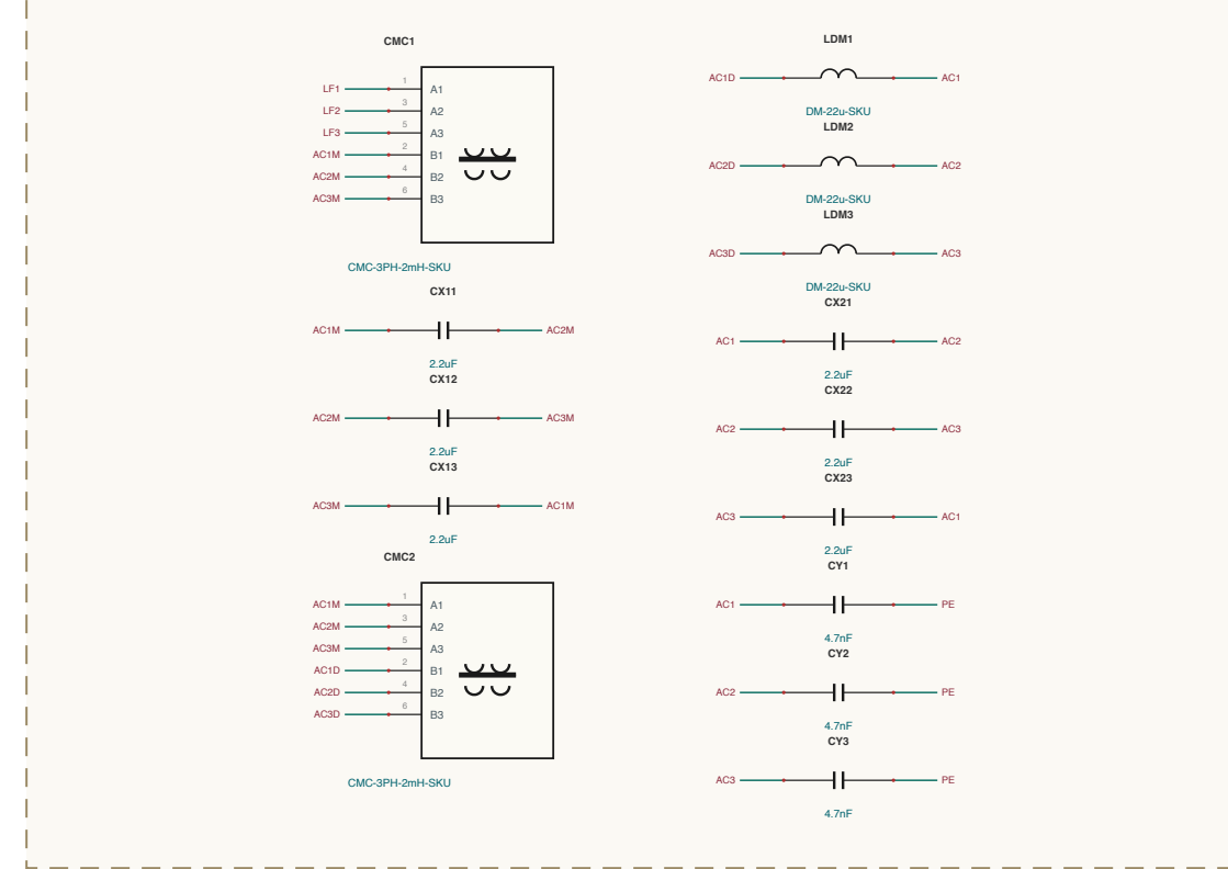
INPUT-EM / EMI-FILTER
