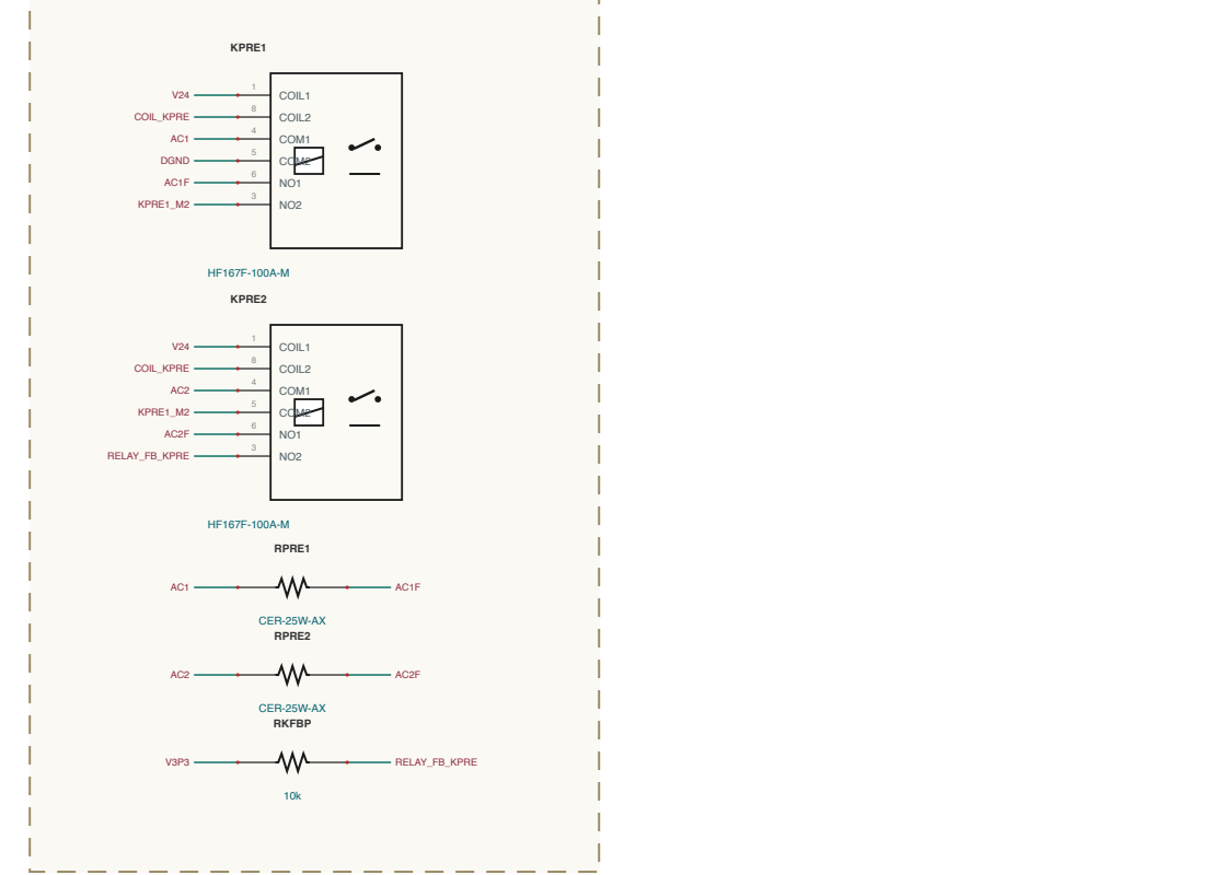
INPUT-EM / PRECHARGE
