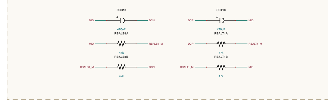
DC-LINK / LINK-BANK-1
