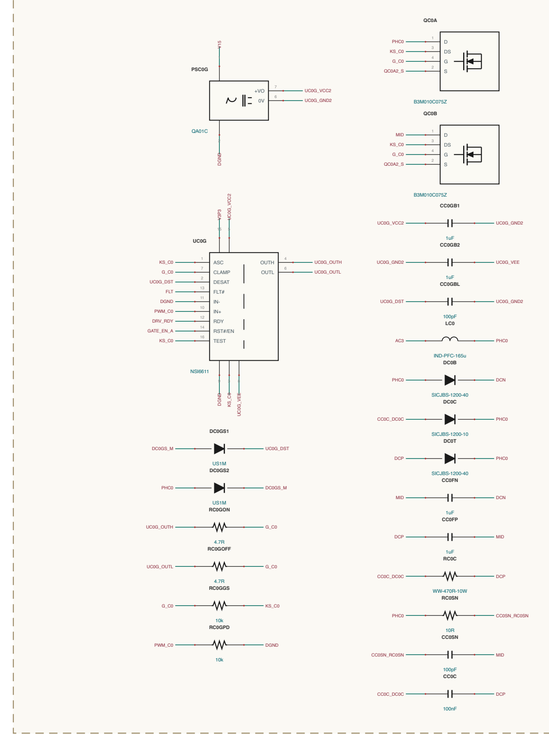
VIENNA-PFC / PHASE-C0
